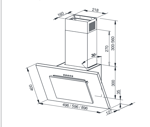
Obr. 2 Rozmery odsávača
