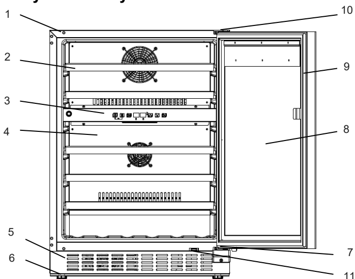
Rys. 2 – Główne części urządzenia.
