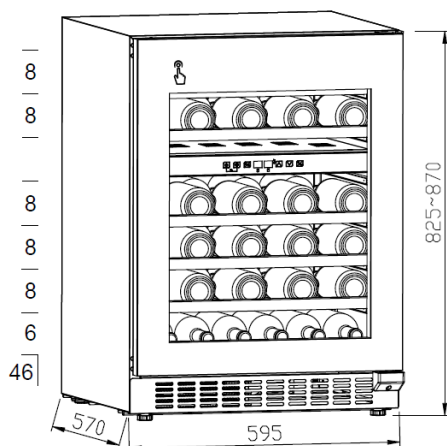
Obr. 4 - Příklad rozmístění 46 standardních lahví Bordeaux o objemu 750 ml.
