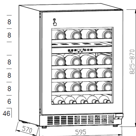
Obr. 4 – Príklad rozmiestnenia 46 štandardných fliaš Bordeaux s objemom 750 ml.
