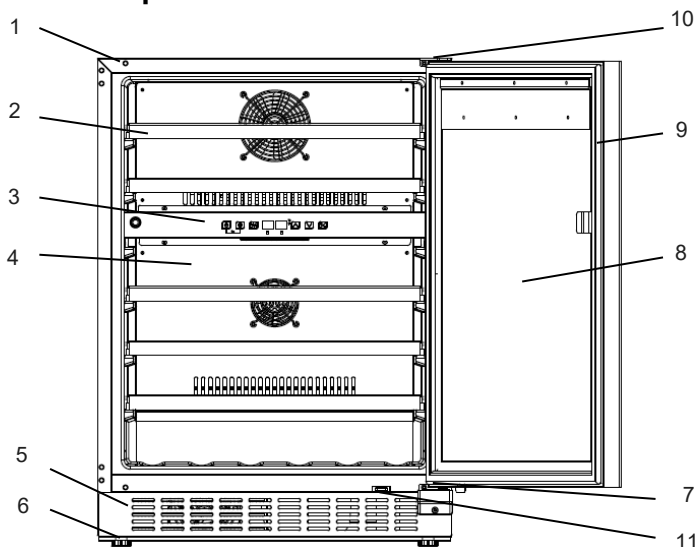
Obr. 2 - Hlavní části spotřebiče.
