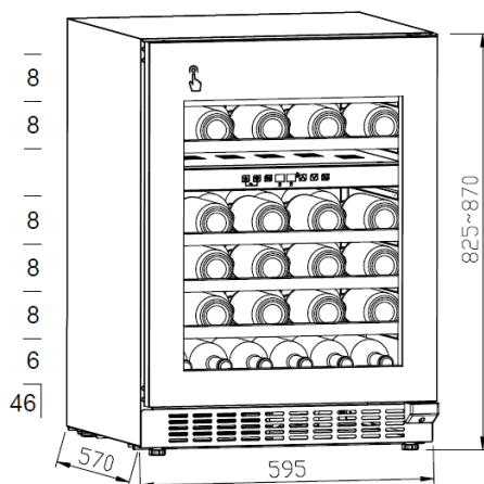
Rys. 4 – Przykład rozmieszczenia 46 standardowych butelek typu Bordeaux o pojemności 750 ml.
