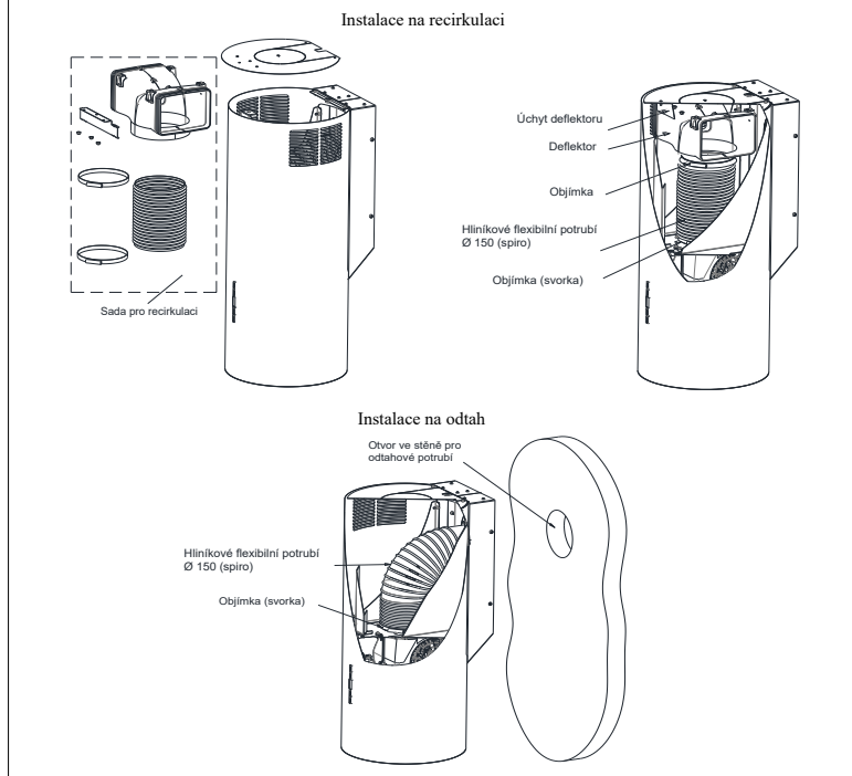
Obr. 3 Možnosti instalace: recirkulace nebo odtah
