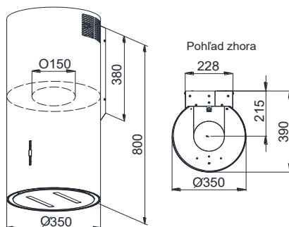
Obr. 2 Rozmery odsávača.
