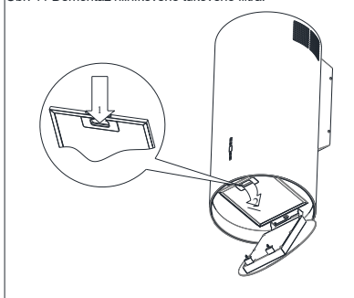
Obr. 11 Demontáž hliníkového tukového filtra.
