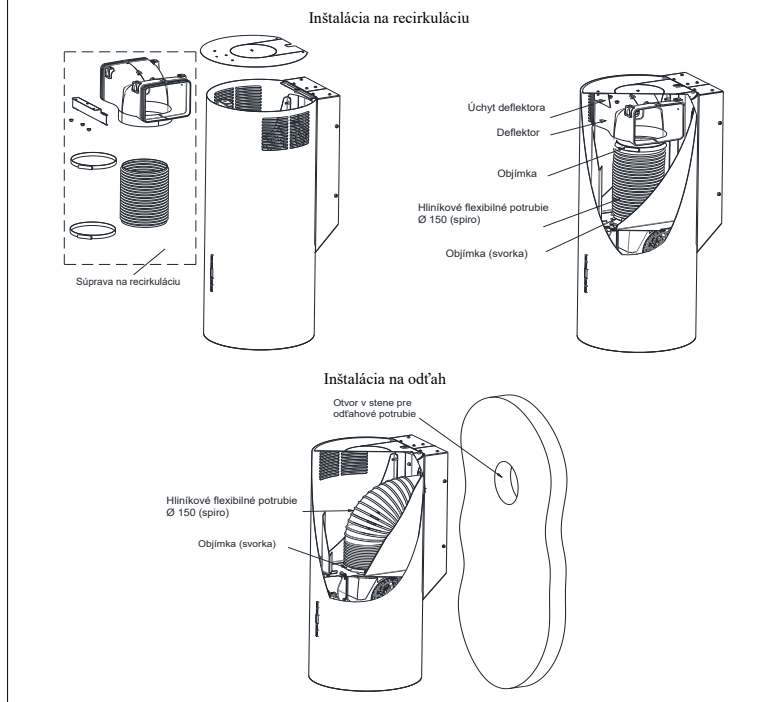
Obr. 3 Možnosti inštalácie: recirkulácia alebo odťah
